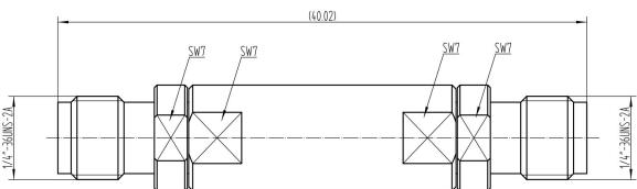
LT-LF-DC-27G-2.92FF
