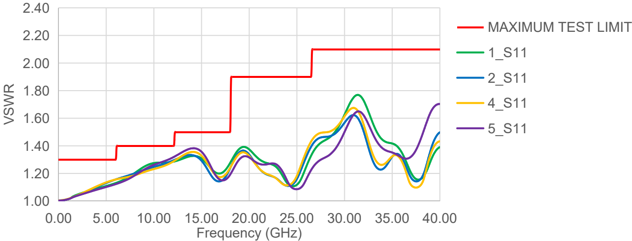
VSWR
