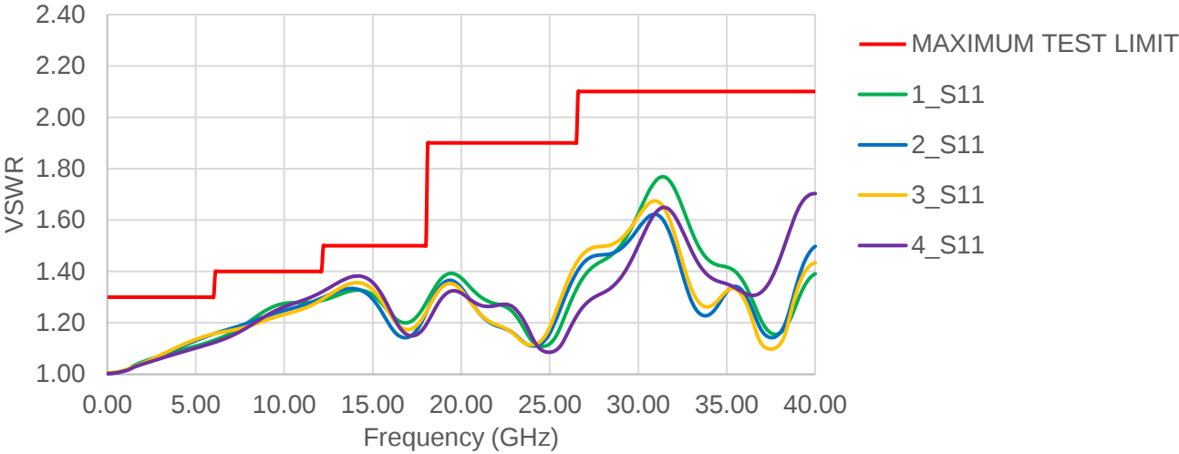
VSWR
