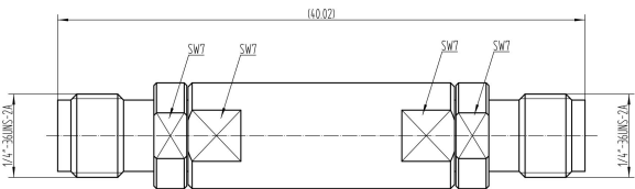
LT-LF-DC-18G-2.92FF
