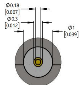
DETAIL B(20:1)
