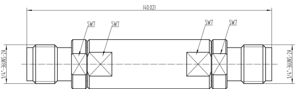
LT-LF-DC-0.8G-2.92FF
