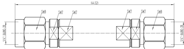
LT-LF-DC-0.8G-2.92MM
